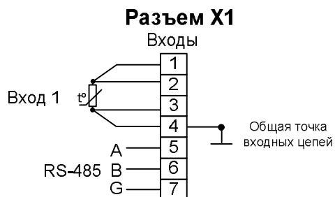
МЕТАКОН-513-Х-ТС-1
