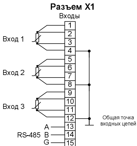
МЕТАКОН-533-Х-ТС-1
