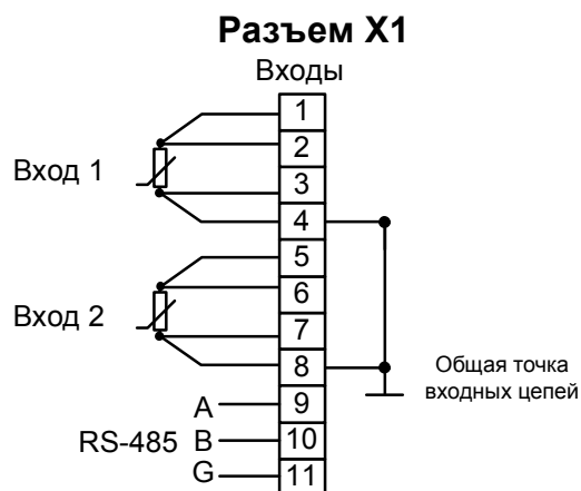
МЕТАКОН-523-Х-ТС-1
